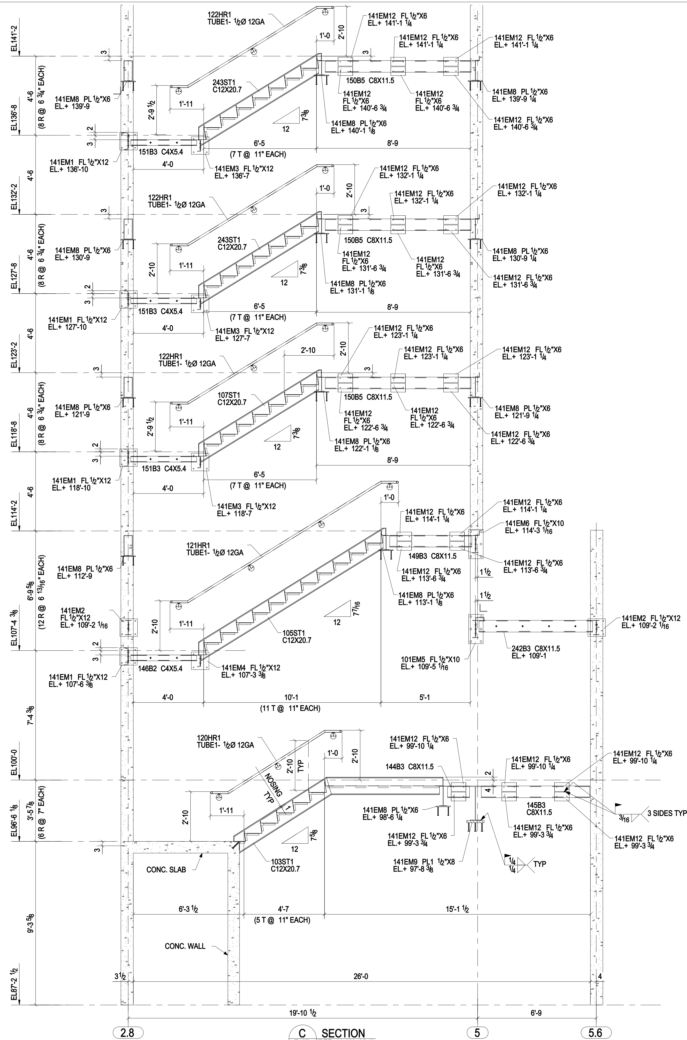
C SECTION E107 (REF-11,13/ A8.4)
